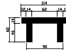
DETALHE DAS VIGAS PRÉ-MOLDADAS (6X) (COMPRIMENTO 10,00 METROS) ESC. 1:20
