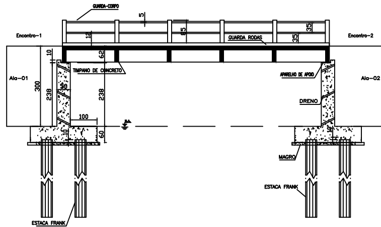
CORTE - B B ESC. 1/50
