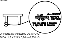
DETALHE DE INSTALAÇÃO DO NEOPRENE EM VIGA ESC. 1:25
