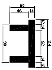
DETALHE DAS VIGAS PRÉ-MOLDADAS (4X) (COMPRIMENTO: 10,00 METROS) ESQ: 1/20
