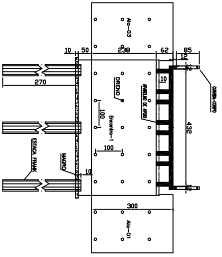
CORTE - A A ESQ: 1/30
