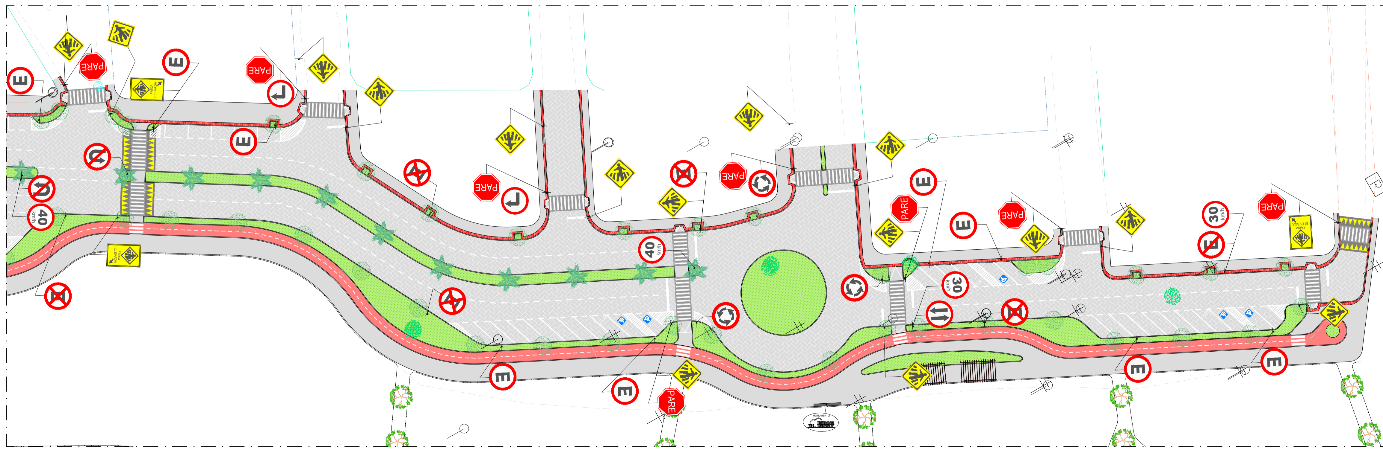
SEÇÃO - 03 ESC.: 1/500
