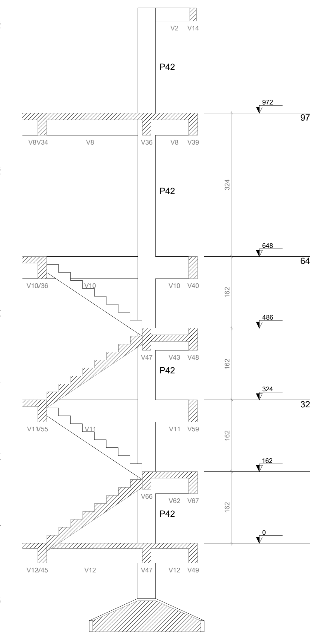
Corte E-E escala 1:50
