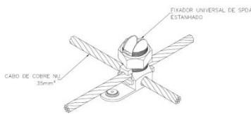
DESENHO 3 - Conexão "X" com fixador universal
