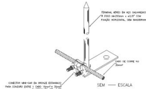
DESENHO 6 - Captor aéreo
