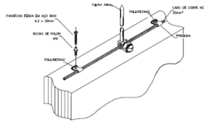
DESENHO 1 - Fixação do captor aéreo na captação
