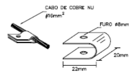
DESENHO 7 - Presilha em latão com furo
