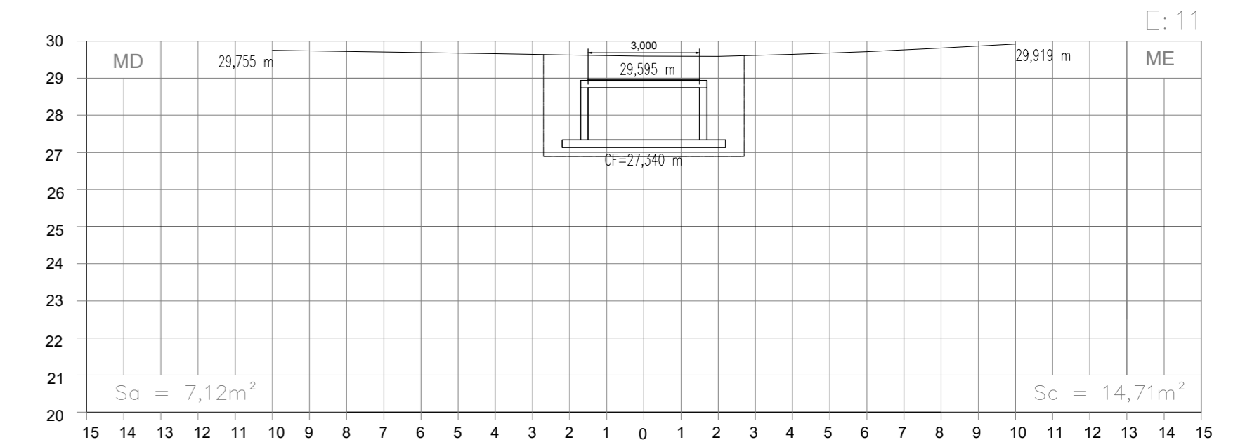
ESC.: H=1/200 V=1/200
