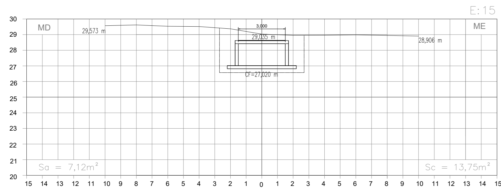
ESC.: H=1/200 V=1/200
