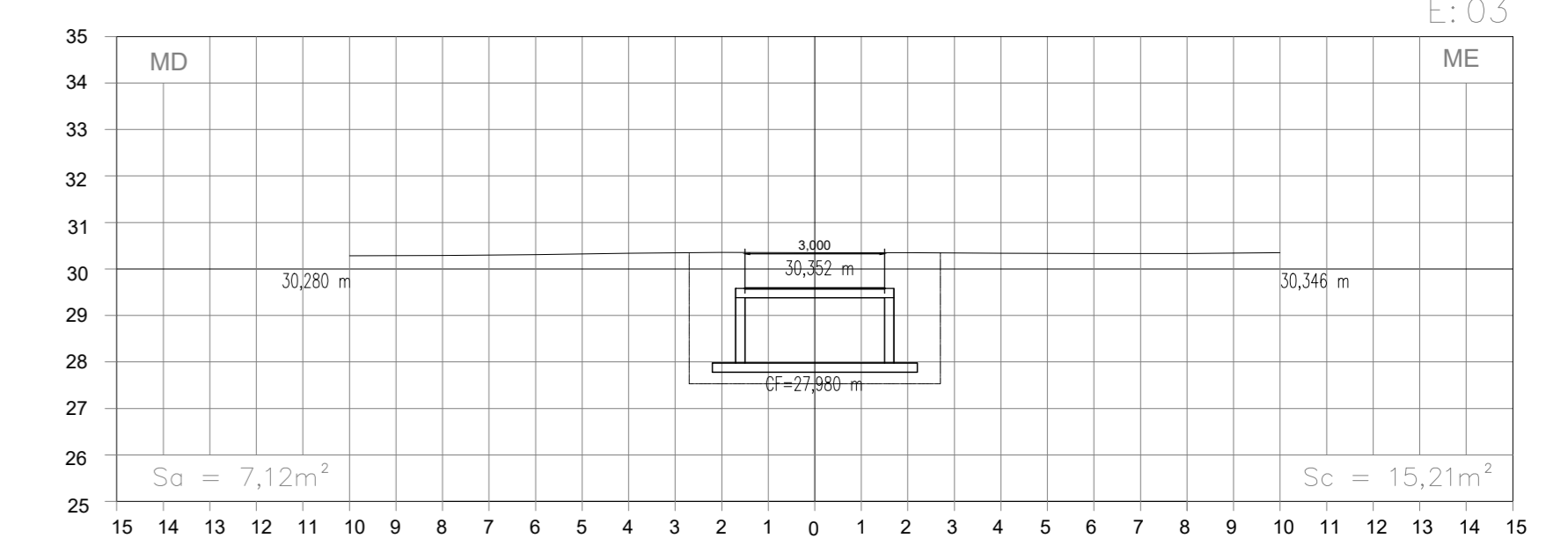
SEÇÕES TRANSVERSAIS ESC.: H=1/200 V=1/200
