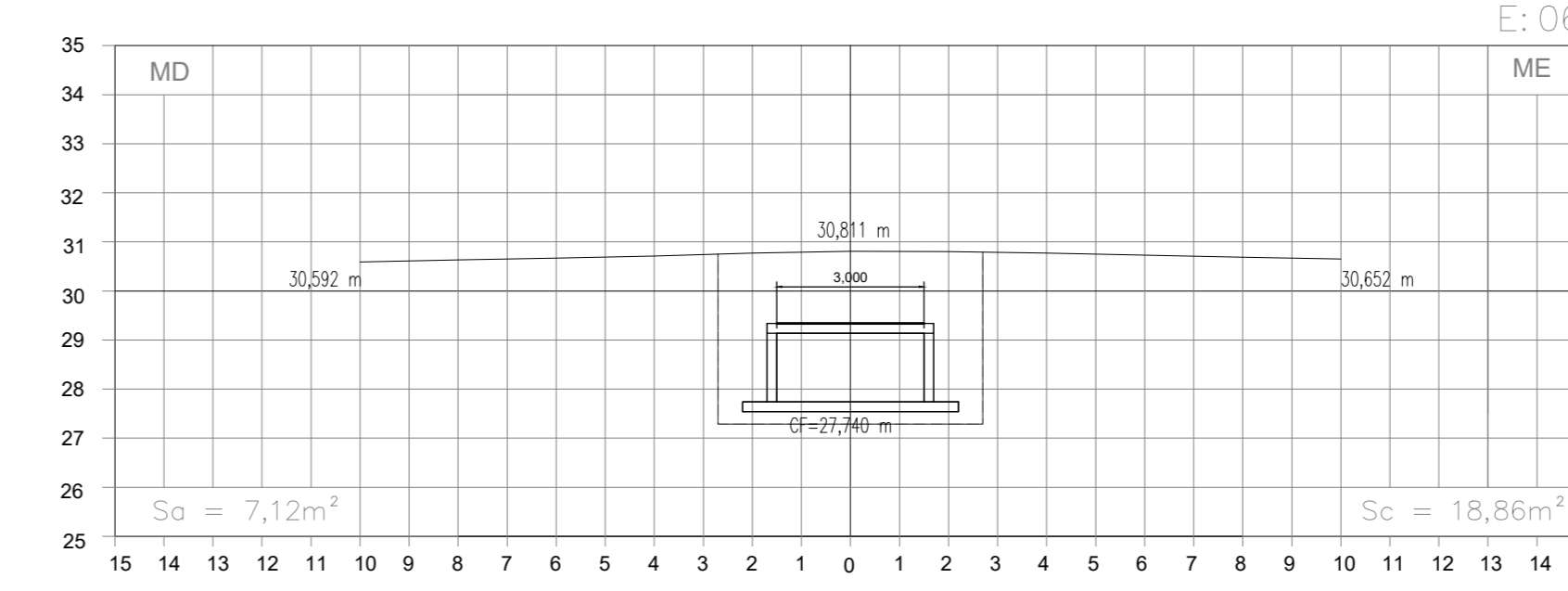
SEÇÕES TRANSVERSAIS ESC.: H=1/200 V=1/200
