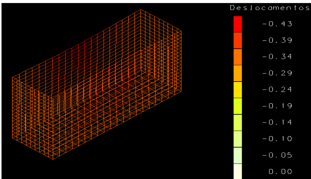
Figura 6 - Deformação
