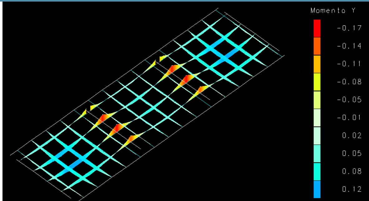
Figura 1 - Momento Fleitor
