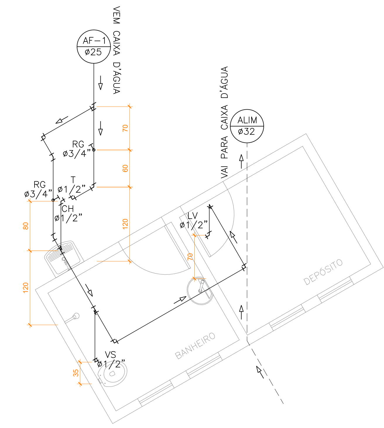
Isométrico água fria - casa de apoio escala 1/50
