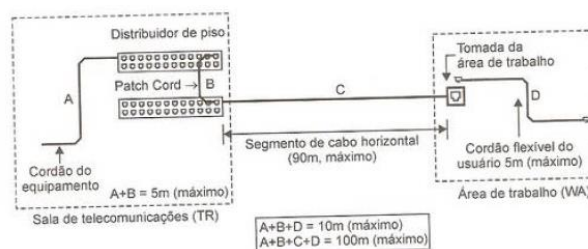
FIGURA 1 – Subsistema de cabeamento horizontal.
