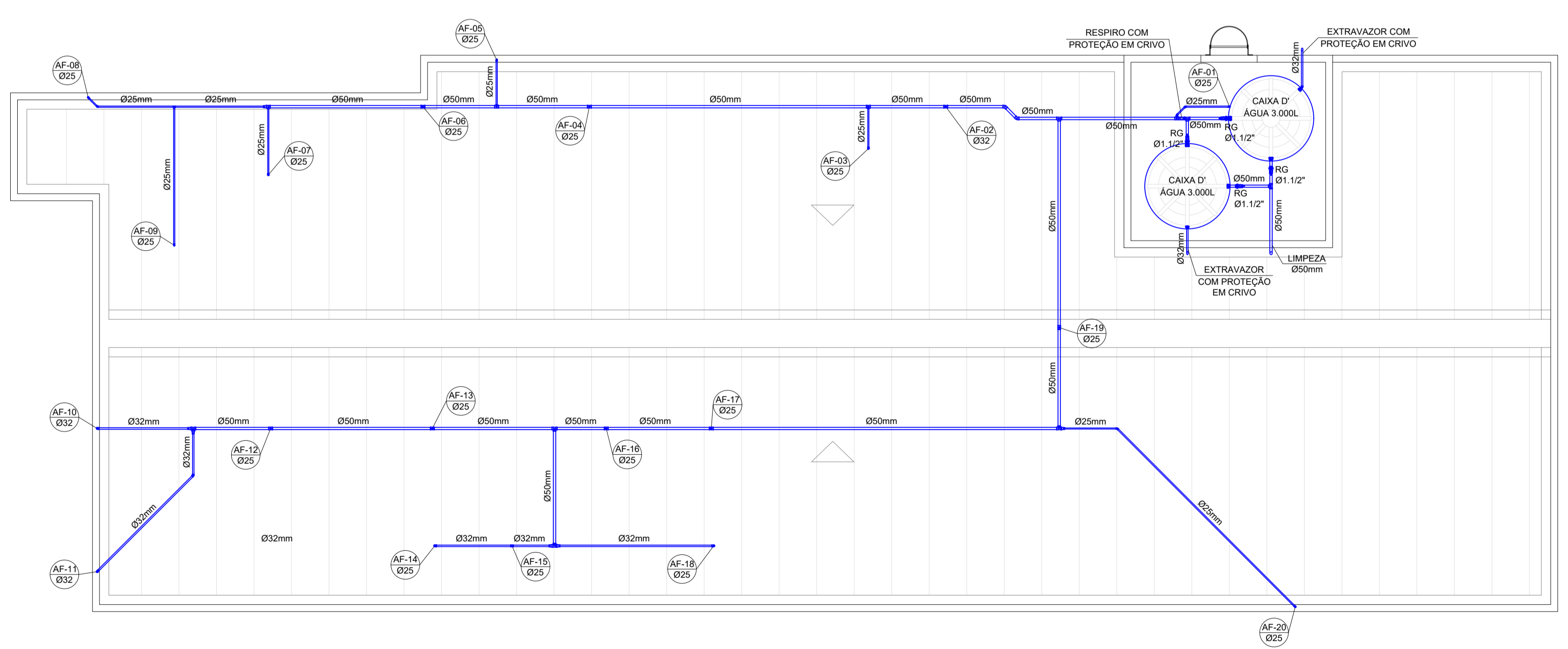
PLANTA BAIXA DE ÁGUA FRIA - COBERTURA ESCALA: 1/75
