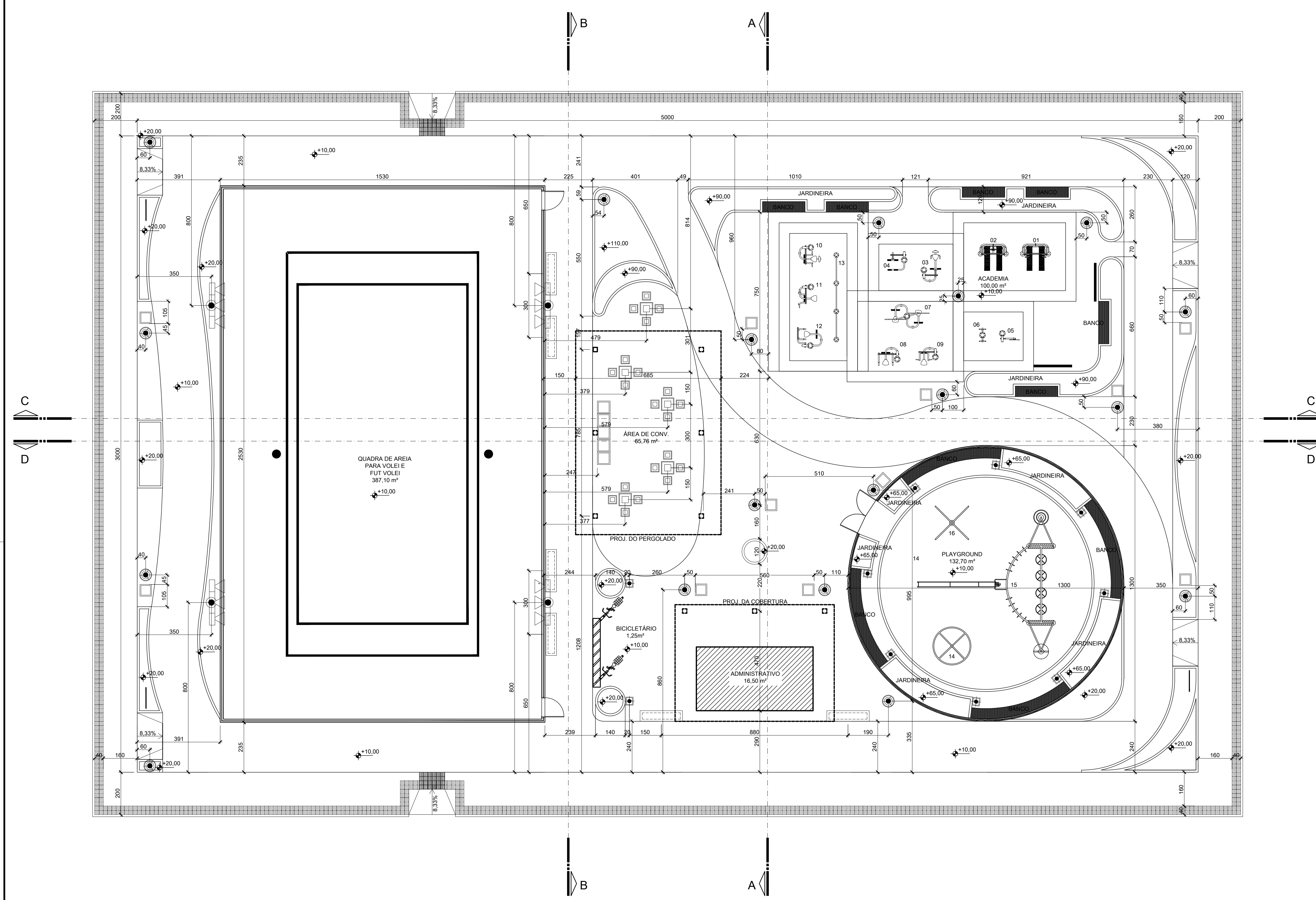
PLANTA DE LOCAÇÃO DE EQUIPAMENTOS - PRAÇA SAUDAVEL - MODELO 1 ESCALA 1:100 ÁREA: 1.500,00m²
