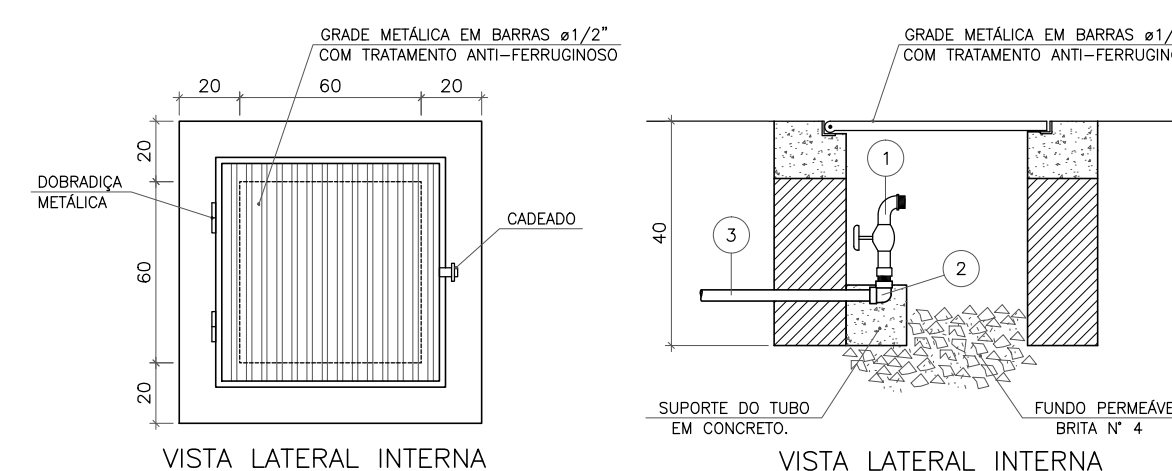
DETALHE DE TORNEIRA DE JARDIM ENTERRADA SEM ESCALA
