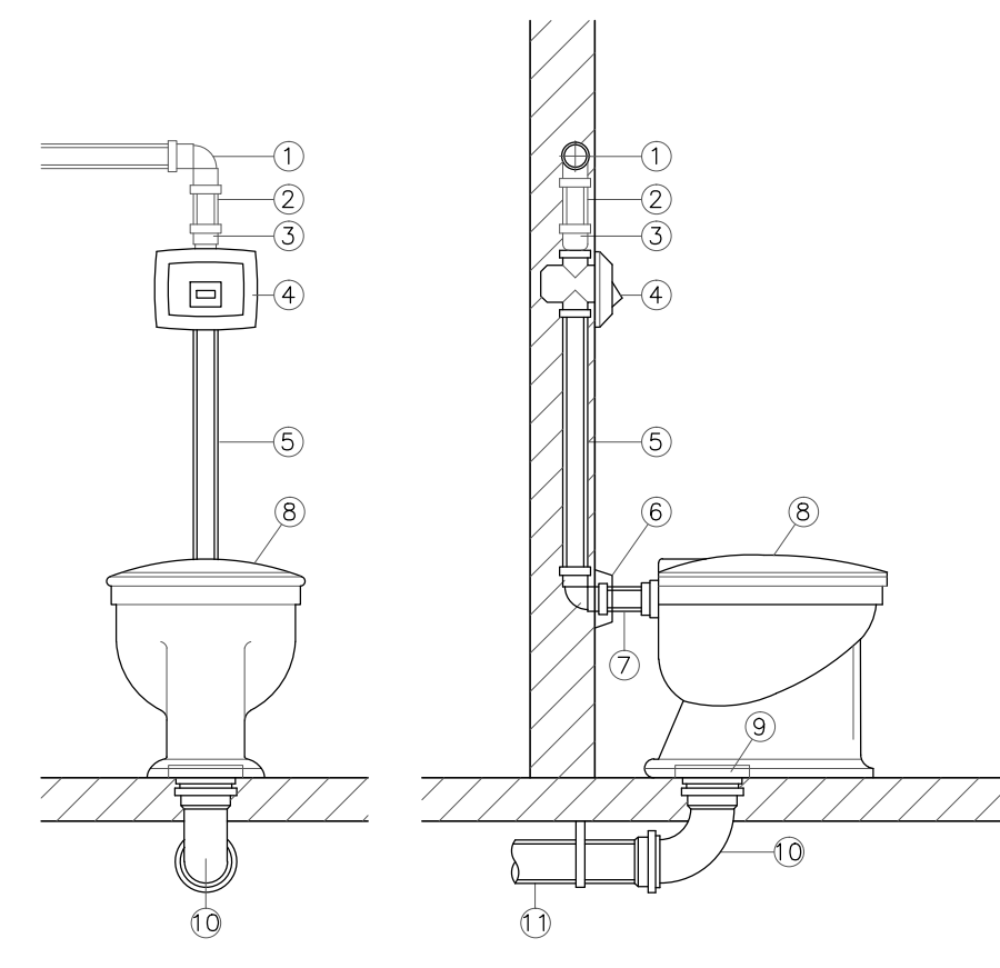
DETALHE DA INSTALAÇÃO VÁLVULA DE DESCARGA PARA VASO SANITÁRIO SEM ESCALA
