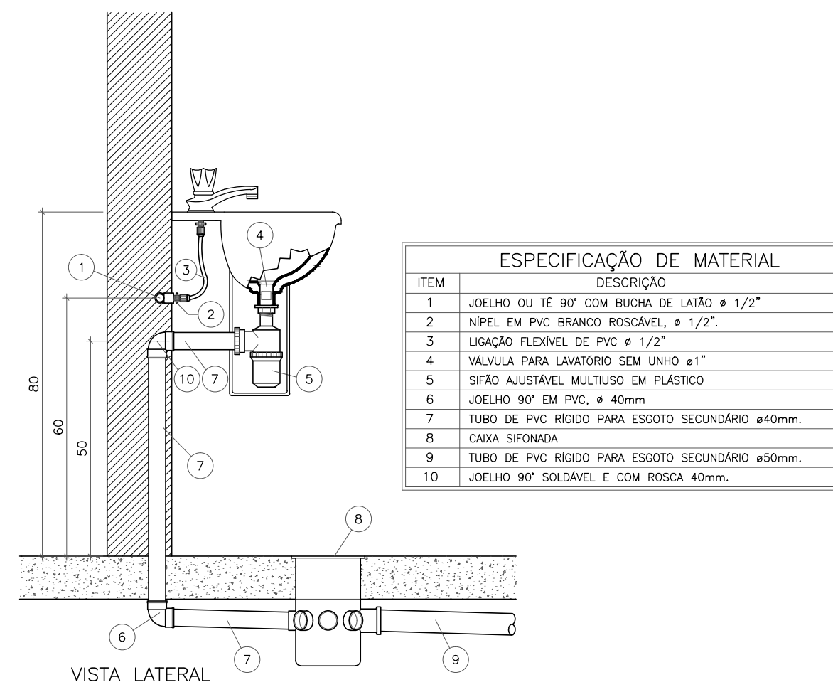
DETALHE DE LAVATÓRIO DE COLUNA SUSPensa SEM ESCALA
