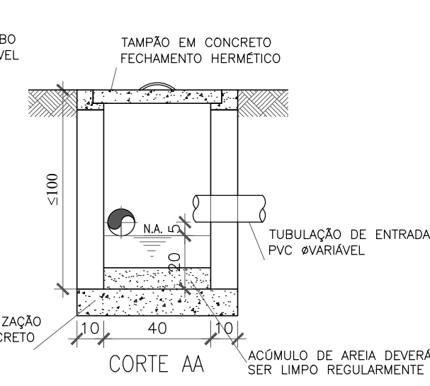
DET. CAIXA DE AREIA (CA)-40x40 ESCALA: 1/20
