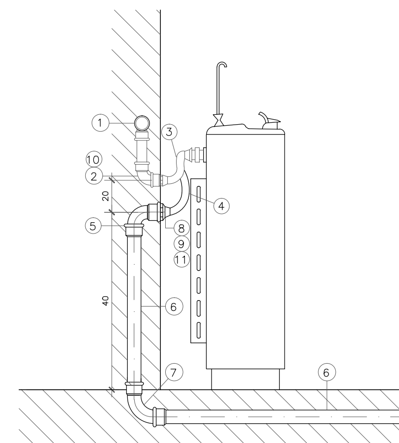
DET. LIGAÇÃO DE BEBEDOURO SEM ESCALA
