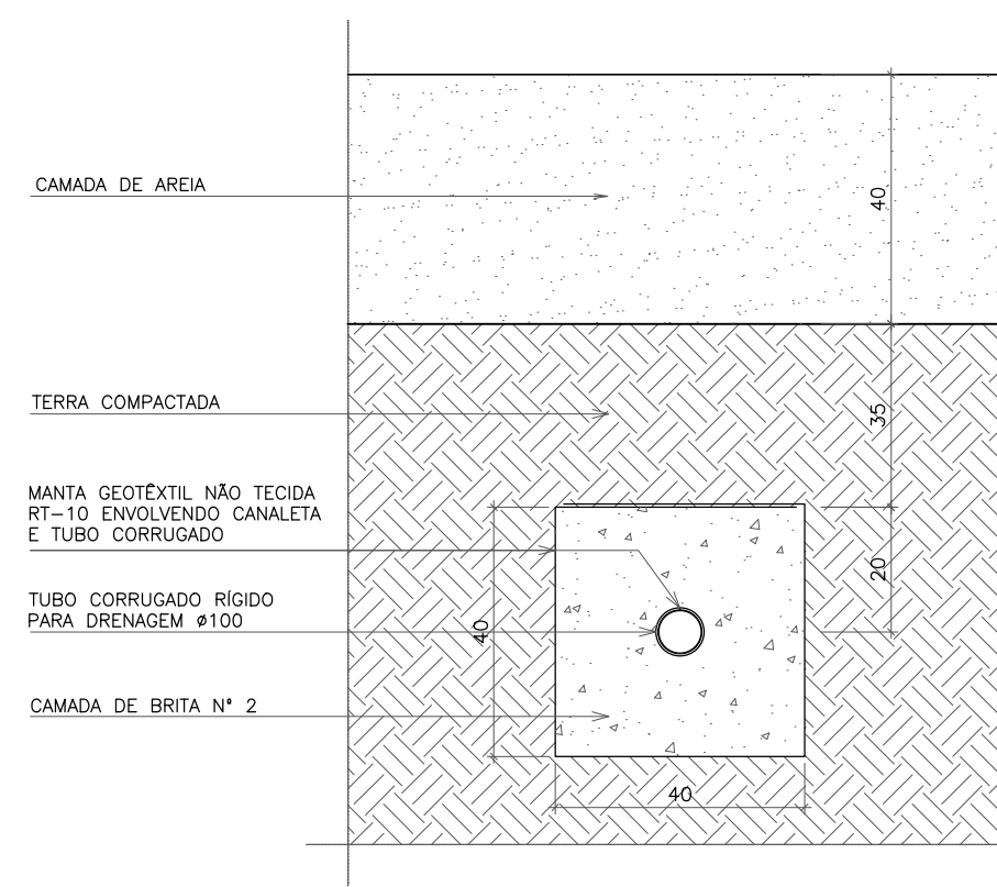
DETALHE INSTALAÇÃO BIDIM SEM ESCALA
