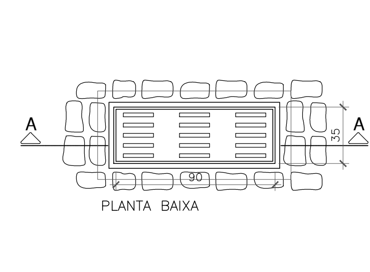
DET. CX. RALO P/ ÁGUAS PLUVIAIS SEM ESCALA
