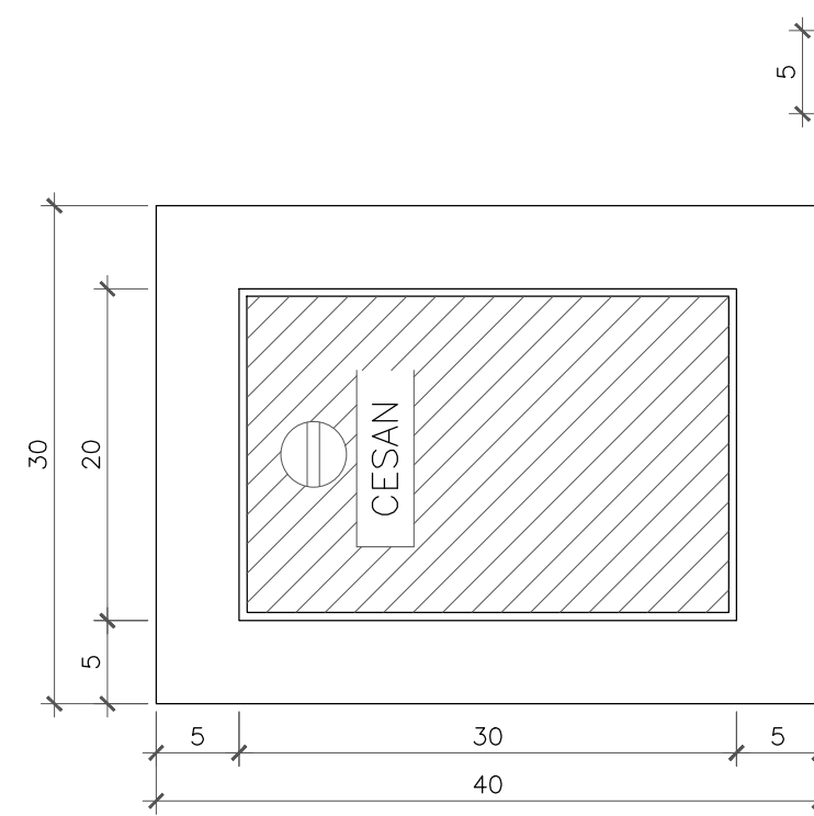
DETALHE HIDRÔMETRO ENTERRADO ESCALA 1/10
