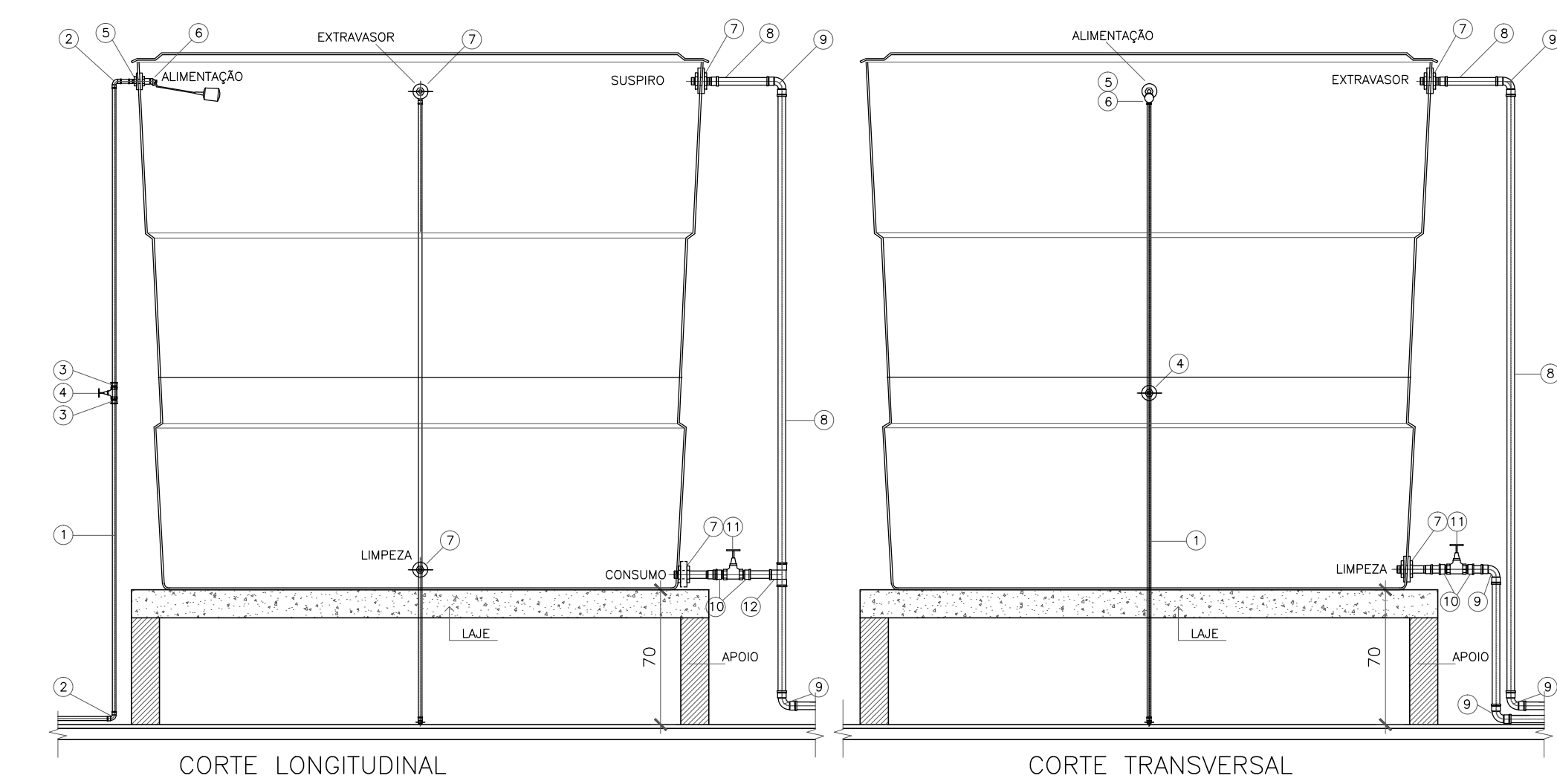
RES. SUPERIOR - 500 LTS. SEM ESCALA
