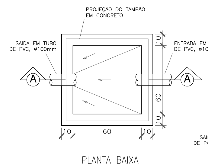
DET. CAIXA DE INSPEÇÃO(CI)-60x60 ESCALA: 1/20
