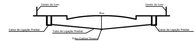
REDE SIMPLES EM VIA
