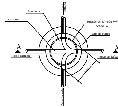
PLANTA BAIXA PV DN 600 ( h < 120 ) DETALHE DO POÇO DE VISITA SEM ESCALA
